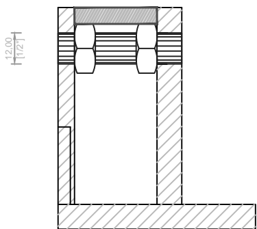
CAÑO DE ALOJAMIENTO DE RULEMANES PARA EJE DE ROTACION
